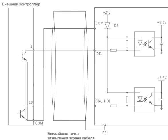
Включение дискретного входа контактом ПЛК
