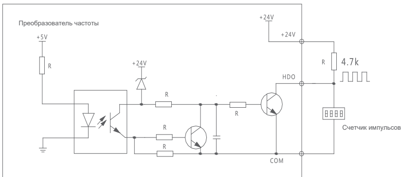
Подключение HDO через внутренний источник питания
